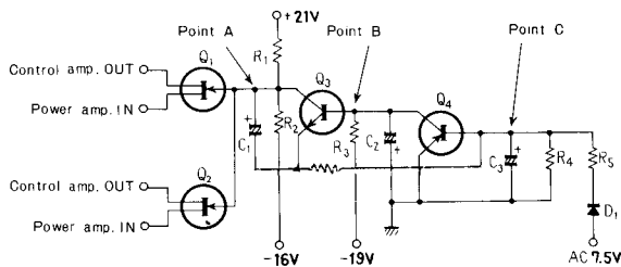
Fig. 5 AF Muting
