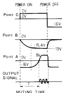
Fig. 5 AF Muting
